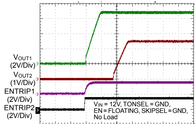
VOUT1 Delay-Start
