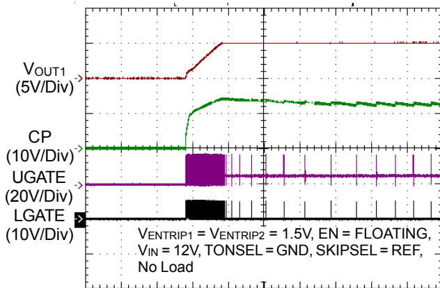
CP Start Up
